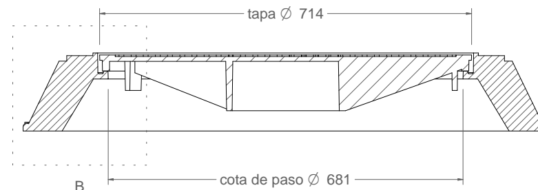
Corte A-A 1:10
