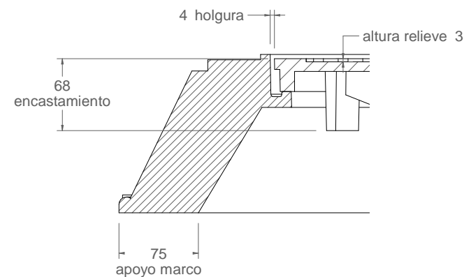
Detalle B
