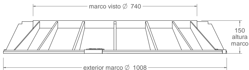
vista alzado 1:10
