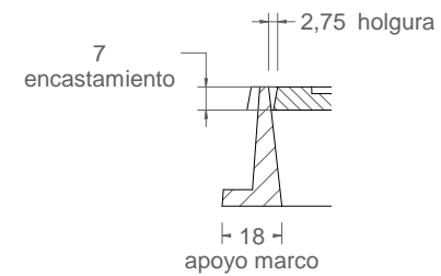
Detalle C
