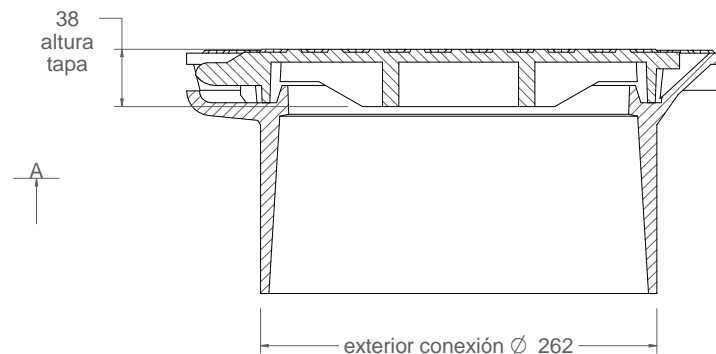
Corte A-A 1:5
