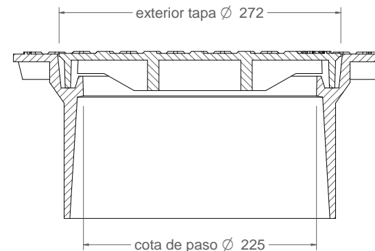
Corte B-B 1:5
