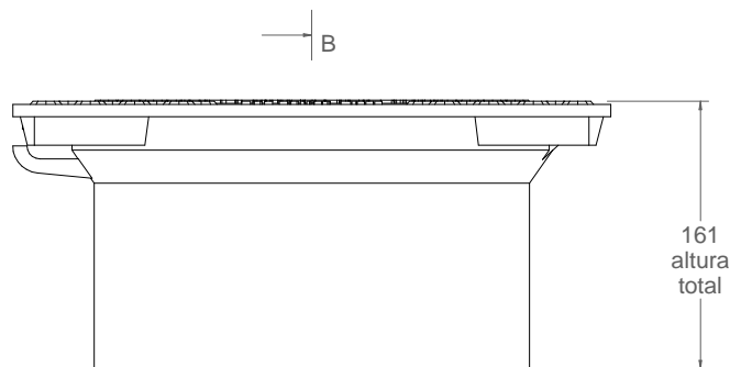
vista alzado 1:5
