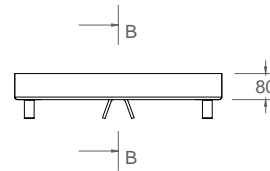
vista alzado 1:20
