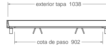
Corte B-B 1:20
