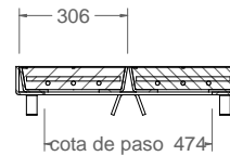
Corte A-A 1:20
