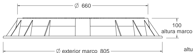
vista alzado 1:10
