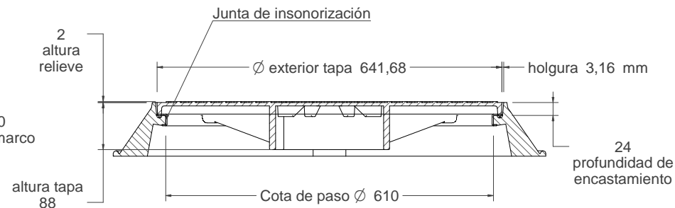
CORTE A-A
