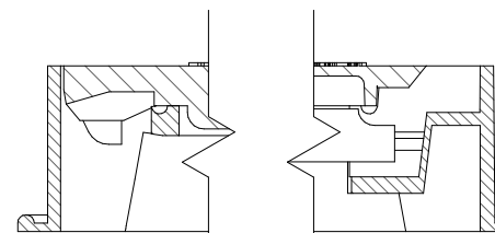
CORTE C-C 1:5
