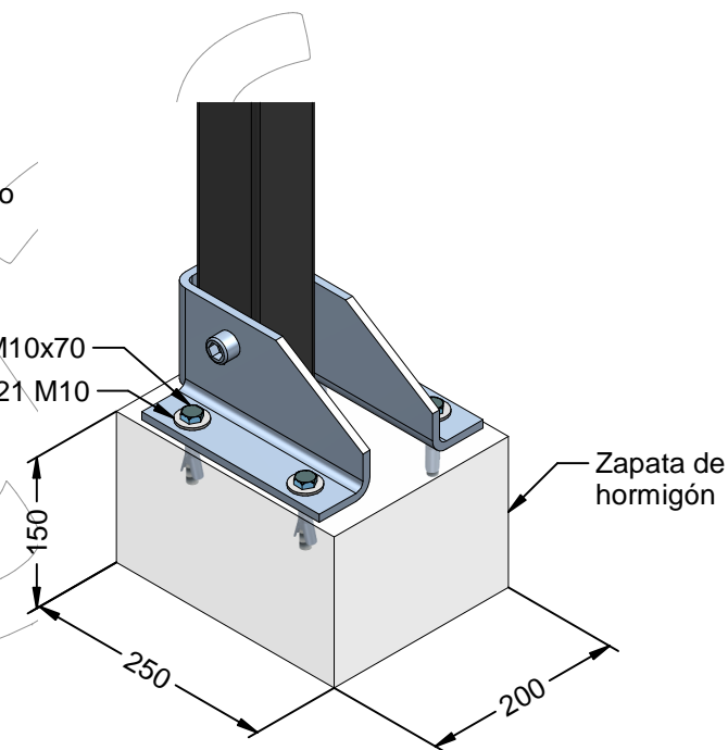
Detalle anclaje
