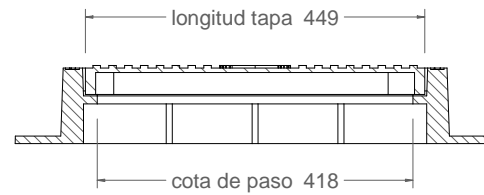
Corte A-A 1:10
