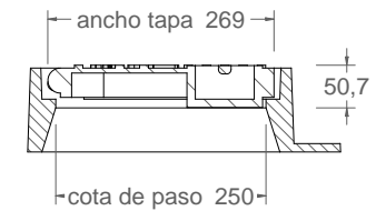
Corte B-B 1:10
