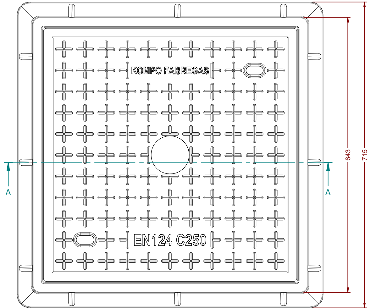
CORTE A-A
