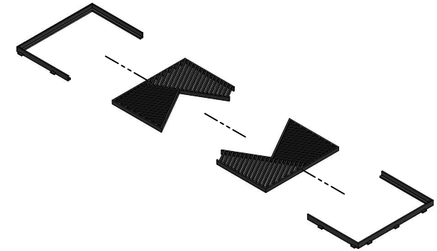
detalle modulación 1:50
