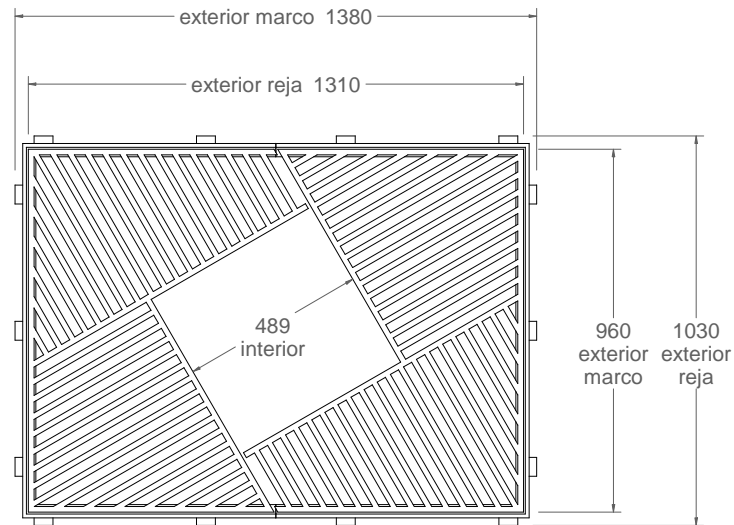
vista en planta 1:20
