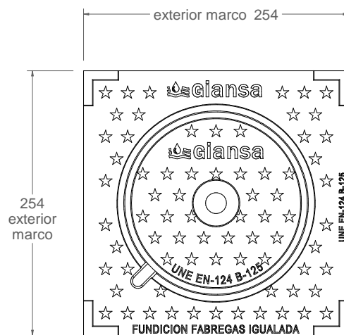
vista en planta 1:5
