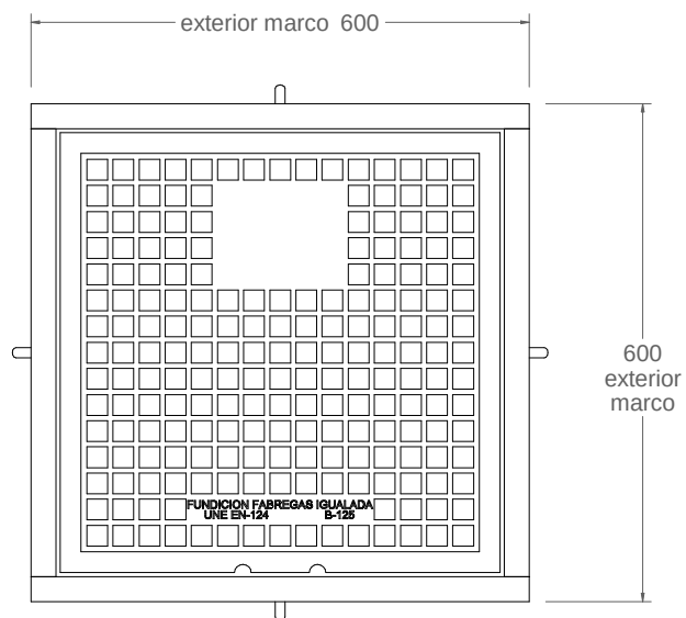
vista en planta 1:10
