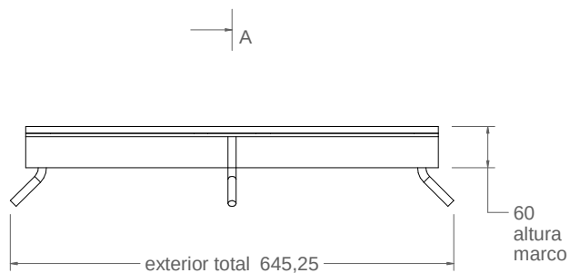
vista alzado 1:10
