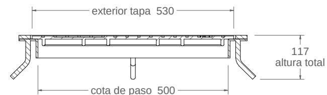
Corte A-A 1:10
