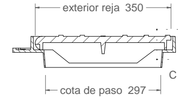
Corte B-B 1:10
