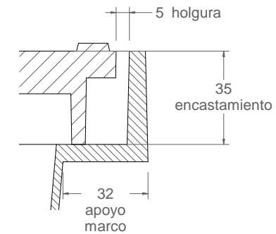
Detalle C
