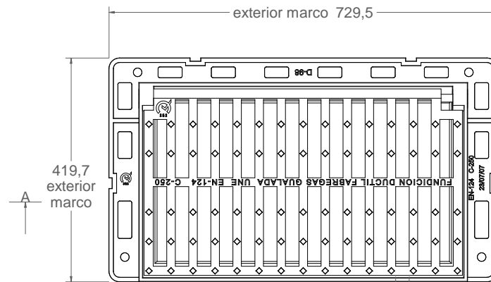
vista en planta 1:10
