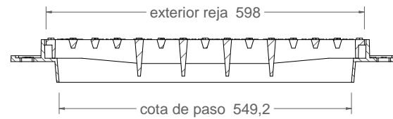
Corte A-A 1:10
