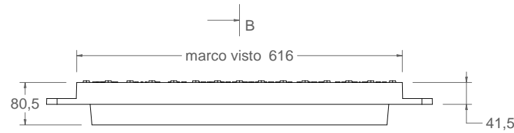
vista alzado 1:10
