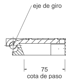
CORTE B-B 1:4
