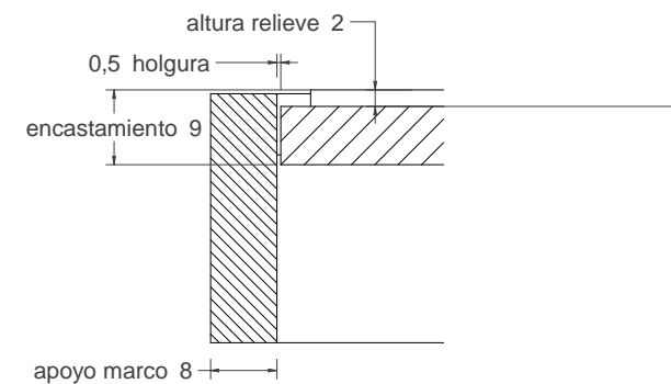
DETALLE C 1:1
