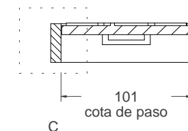
CORTE A-A 1:4
