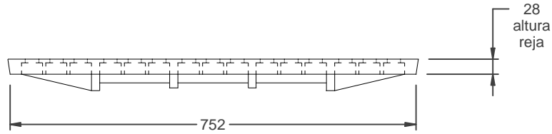
vista alzado 1:10
