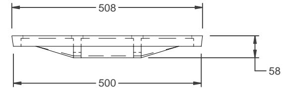
vista lateral 1:10
