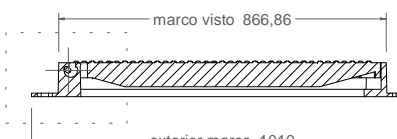
CORTE D-D 1:20
