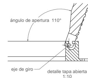
DETALLE F 1:10
