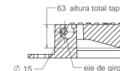
DETALLE E 1:10
