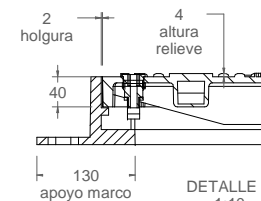
DETALLE C 1:10
