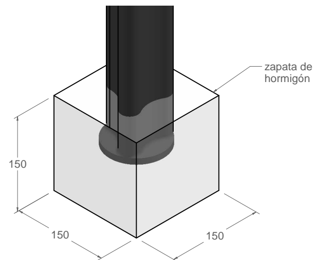
detalle anclaje 1:5
