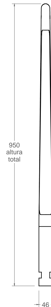
vista alzado
