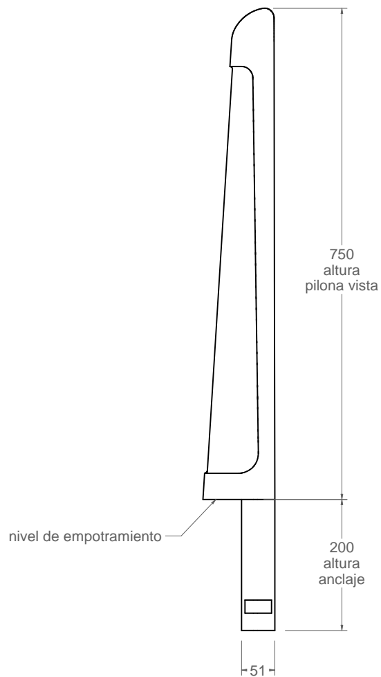
vista lateral
