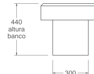
vista lateral 1:20
