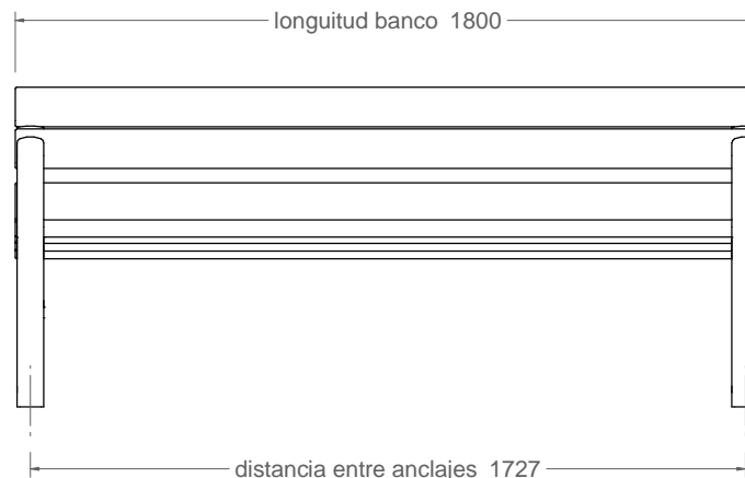
vista alzado 1:20
