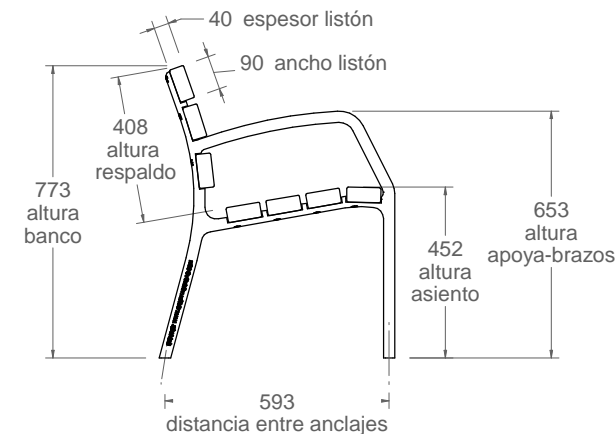
vista lateral 1:20
