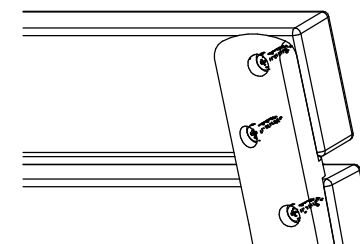
Detalle anclaje listones 1:5
