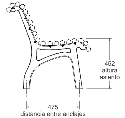
vista lateral 1:20
