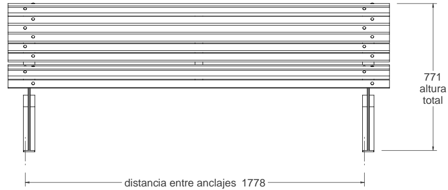
vista alzado 1:20
