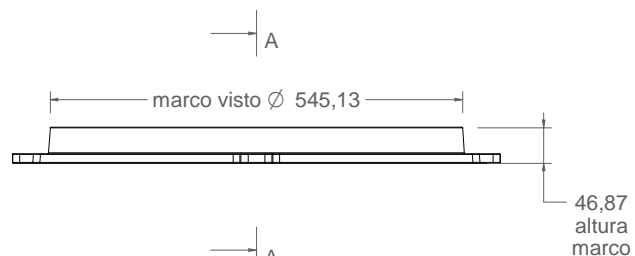
vista alzado 1:10
