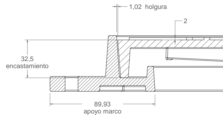
Detalle B 1:2
