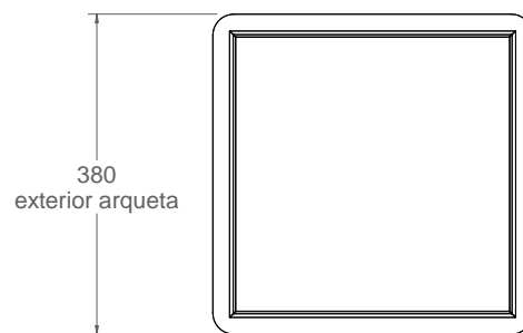
Vista en planta 1:10
