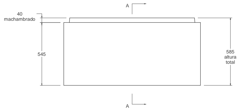
vista alzado 1:20
