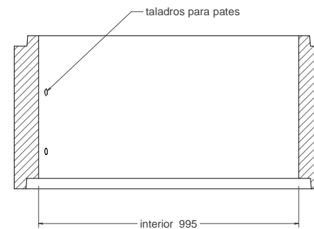
Corte A-A 1:20
